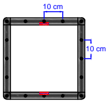
1. Montaje Frontal
