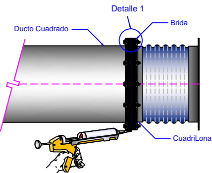
2. Montaje Lateral
