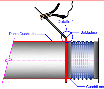
2. Montaje Lateral
