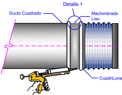
2. Montaje Lateral
