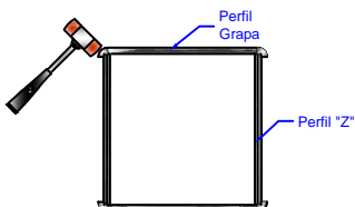
1. Montaje Frontal
