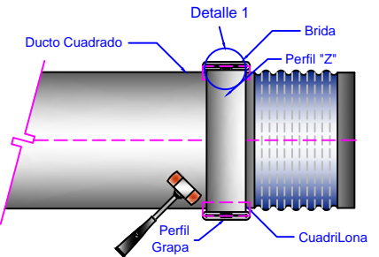
2. Montaje Lateral
